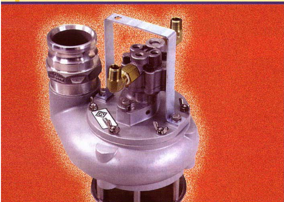
A FAIRMONT 3" zagyszivattyú mindössze 11 kg. Max. emelési magassága 33 m, folyadékcszállítása 1900 l/perc. Önfelszívó, minden elképzelhető anyagot szállít.
